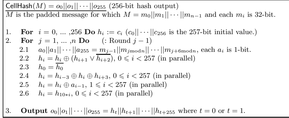
Fig. 1. CellHash Algorithm.
